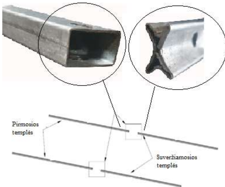
Pav. 11 Pirmųjų templių jungimas su suveržiamosiomis templėmis
