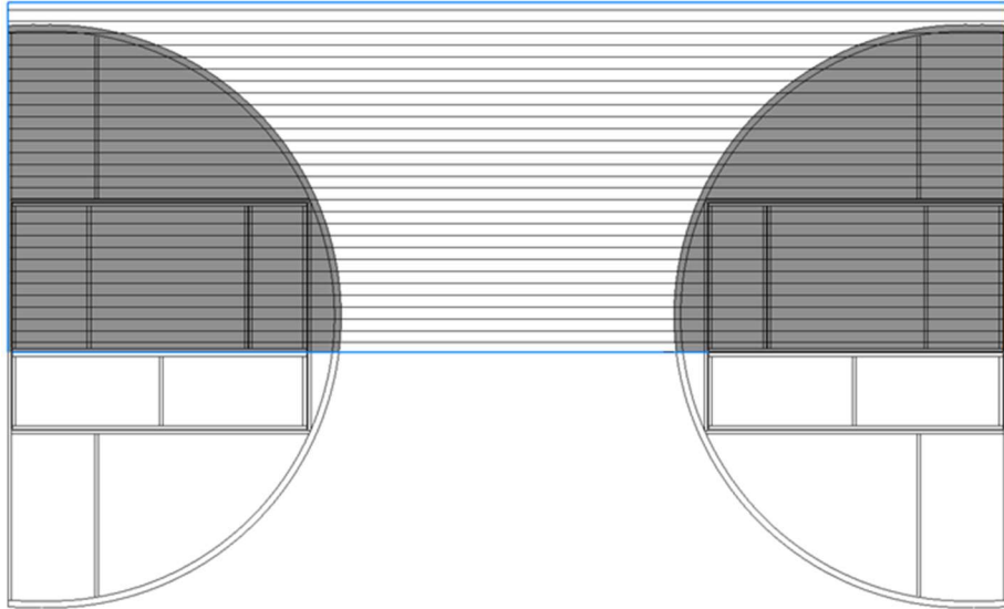
Pav. 2 Polikarbonato montavimo schema šiltnamio galuose
