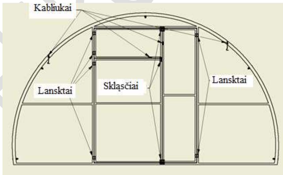
Pav. 9 Kabliukų, skląščių, lankstų tvirtinimo vietos ant šiltnamio arkos
