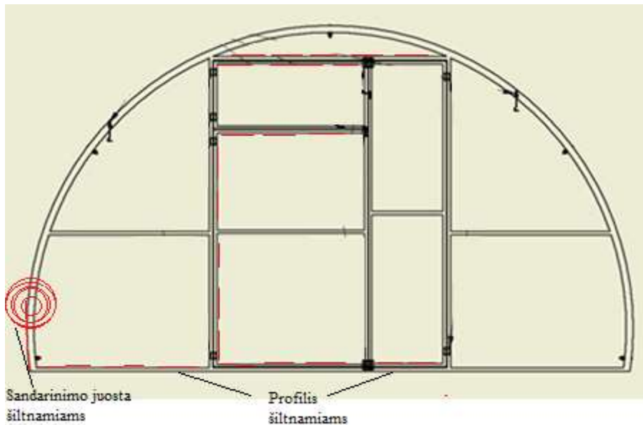
Pav. 8 Polikarbonato dangos montavimas ant šiltnamio rėmo
