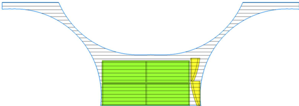
Pav. 4 Polikarbonato montavimo schema likusioms arkų dalims
