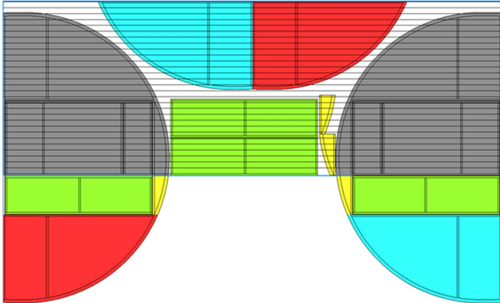
Pav. 1 Polikarbonato lapo (6x2,1 m) išdėstymas šiltnamio priekinei bei galinei arkoms uždenkti
